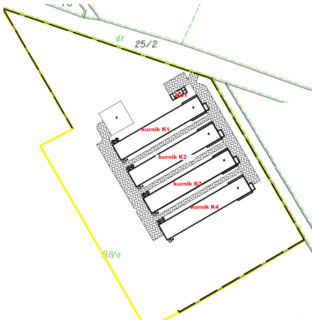
Rysunek nr 3.2.2-1 Lokalizacja planowanych budynków na terenie Fermi
